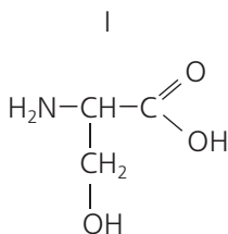
серин
