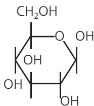
1 β-D-глюкоза
