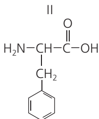
фенилаланин
