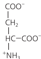
3 аспарагиновая кислота
