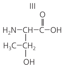
треонин
