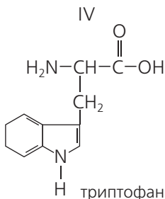
триптофан
